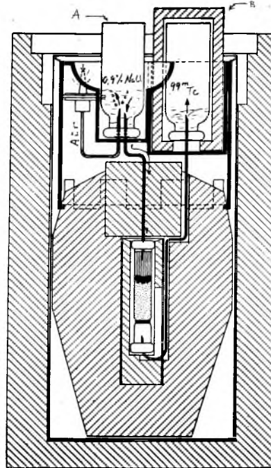
Şekil 1: MON. TEK Mo 99 /Tc 99m JENERATÖR sağım şeması
