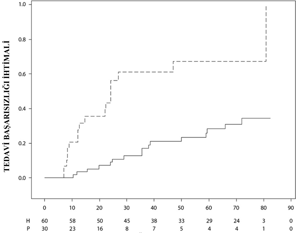
Şekil 2: Pediyatrik üveit çalışmasında tedavi başarısızlığına kadar geçen süreyi özetleyen Kaplan-Meier Eğrileri
